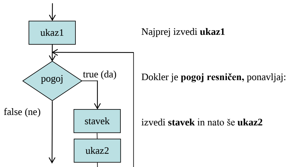
Slika 19: Diagram poteka za for zanko
